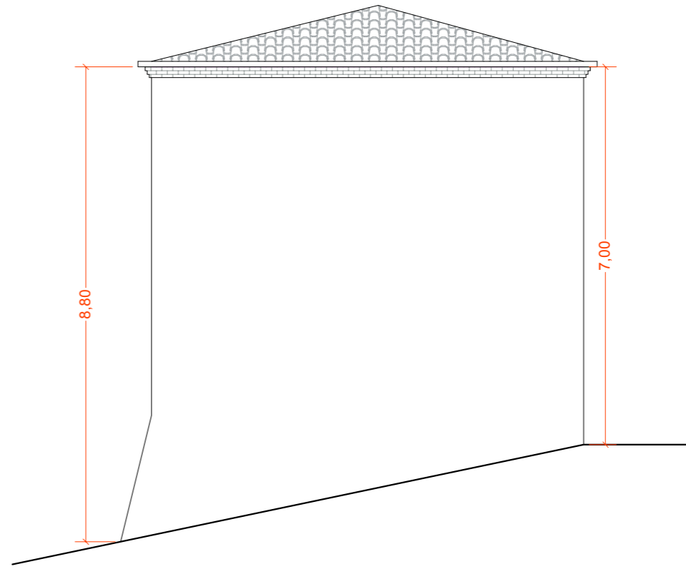
PROSPETTO NORD
